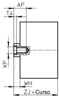
Rosca Fêmea
